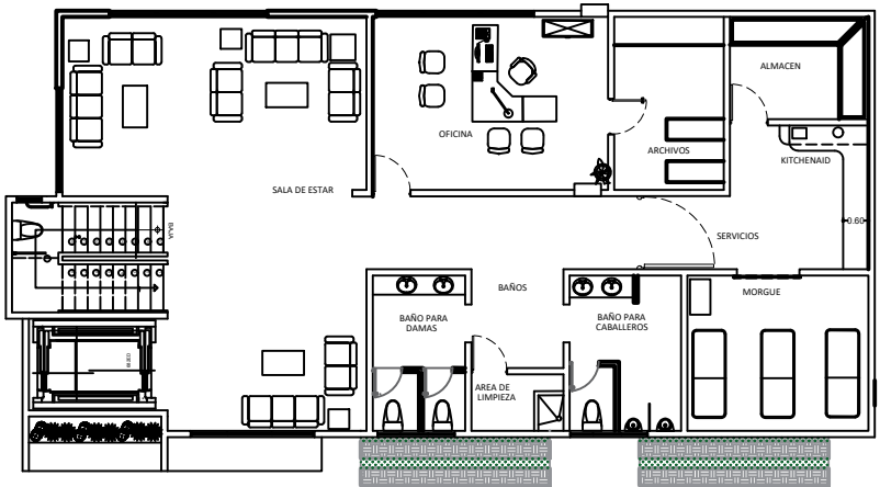
PLANTA ARQUITECTONICA FUNERARIA 2DO NIVEL ESC:1:100
