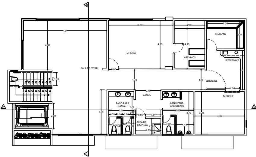
PLANTA DIMENSIONADA FUNERARIA 2DONIVEL ESC:1:100
